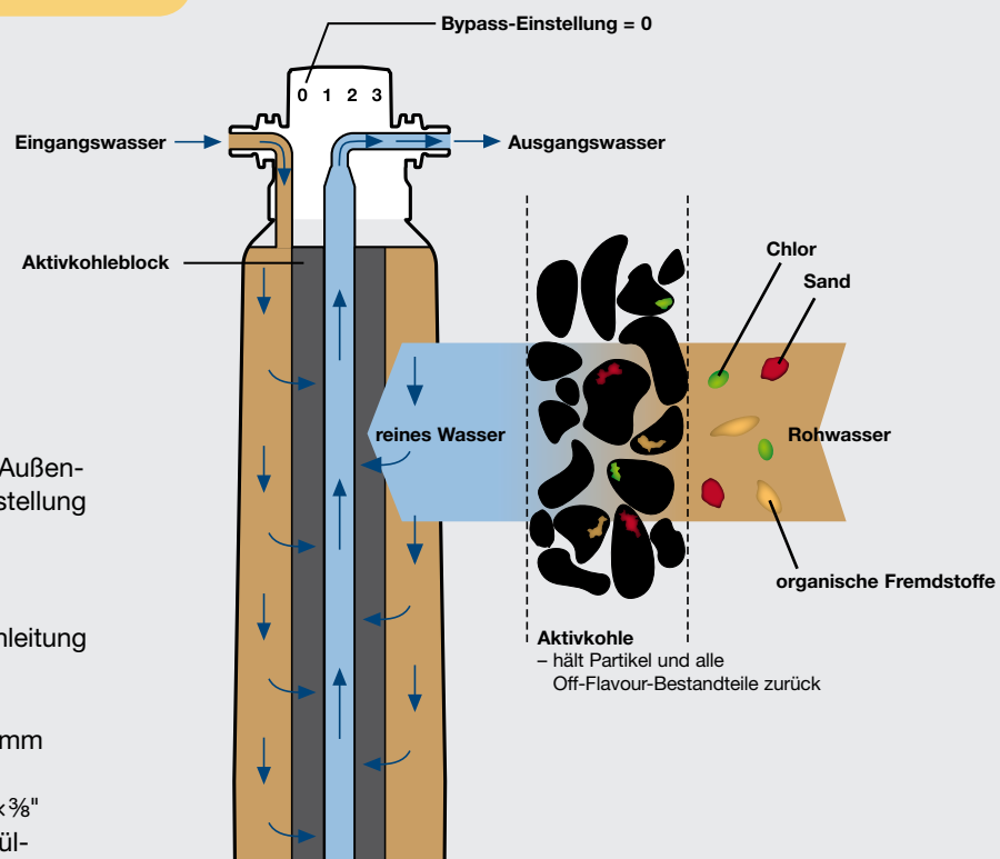
Aufbau einer besttaste-Filterkerze
