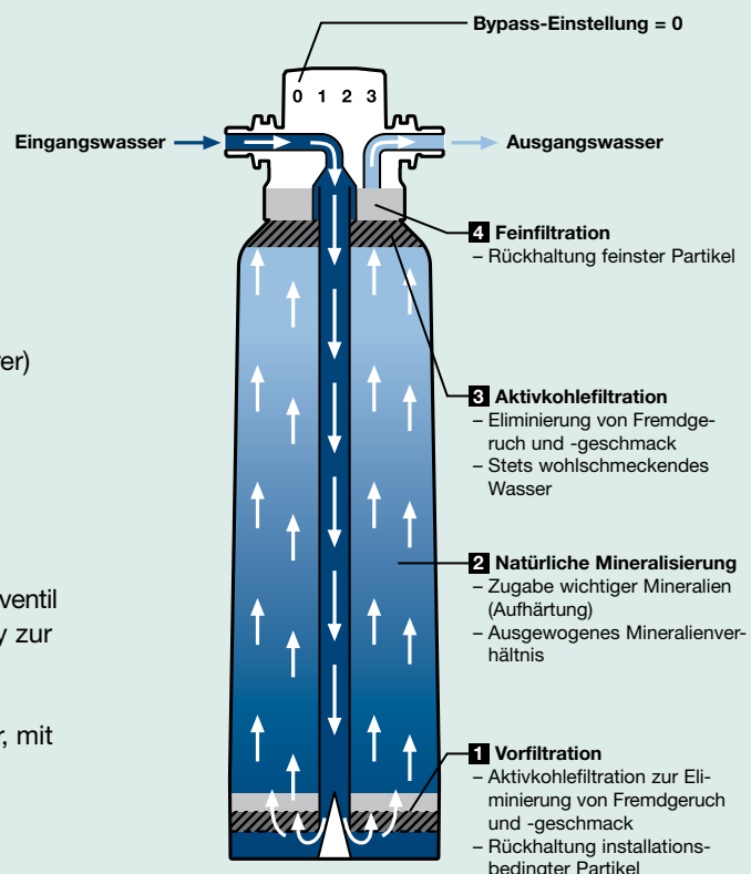
Aufbau einer bestmin-Filterkerze
