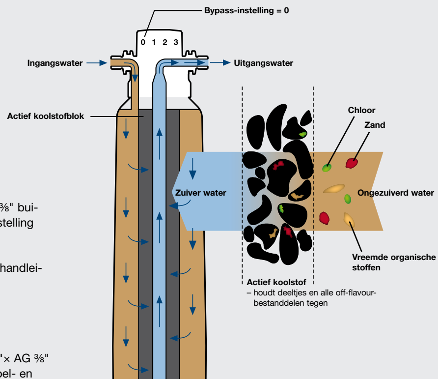
Opbouw van een besttaste-filterpatroon
