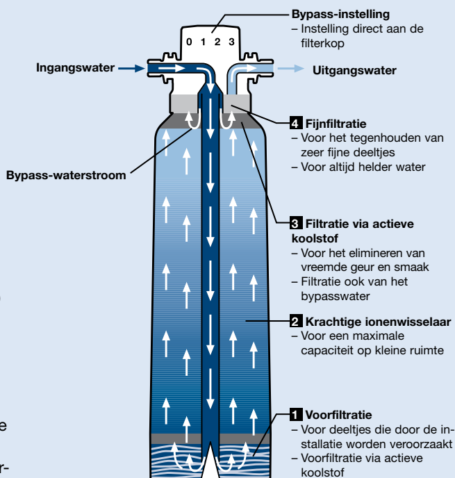
Opbouw van een bestmax PREMIUM filterpatroon
